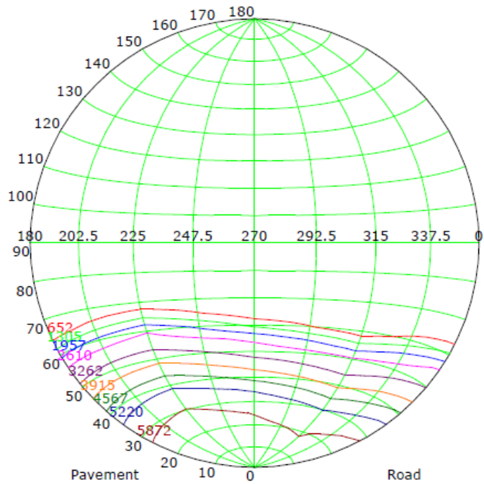
Imax (100%): 6524 cd
